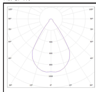
配光曲線
